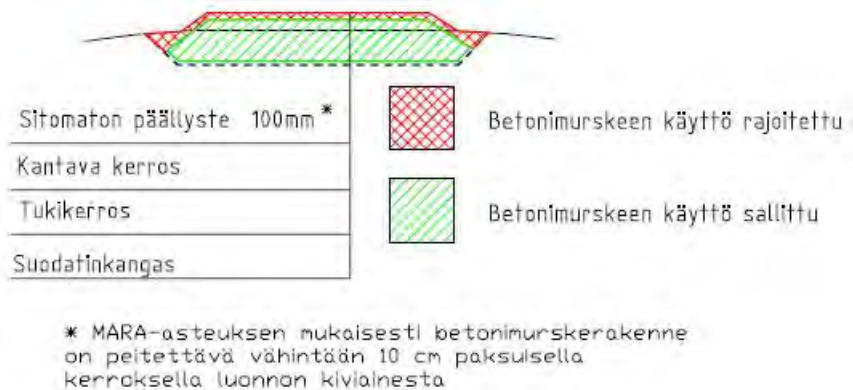
Kuva 1 Betonimurskeen käyttömahdollisuuksia ja -rajoituksia raitin poikkileikkauksessa.
